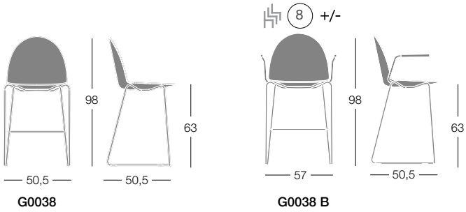
SGABELLO IMPILABILE A SLITTA H. 63 CM / STACKING SLED STOOL H. 63 CM / TABOURET EMPILABLE BASE TRINEAU H. 63 CM / BARHOCKER STAPELBAR SITZHÖHE H. 63 CM
