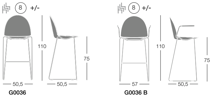
SGABELLO IMPILABILE A SLITTA H. 75 CM / STACKING SLED STOOL H. 75 CM / TABOURET EMPILABLE BASE TRINEAU H. 75 CM / BARHOCKER STAPELBAR SITZHÖHE H. 75 CM
